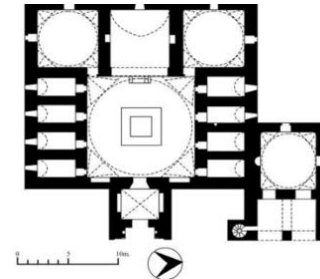
شكل رقم (٥): مسقط أفقي لمدرسة انجه منارة لي بقونية والمسجد الملحق بها من قبة وتتقدمها سقيفة (عن: Hillenbrand)
