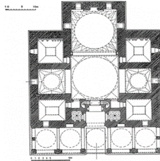
شكل رقم (٣): مسقط أفقي لجامع بايزيد يلدريم في بورصة يمثل طراز بورصة الثالث (عن: أصلان آبا)
