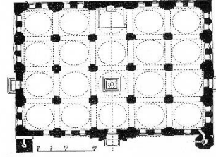
شكل رقم (٢): مسقط أفقي ومنظور لأولو جامع في بورصة يمثل طراز بورصة الثاني (عن: Hillenbrand ، Ünsal، Bahçet)
