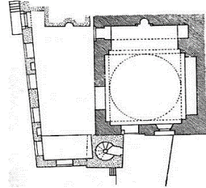
شكل رقم (٩): مسقط أفقي لجامع كتخدا العزب بالقاهرة يوضح زيادة مساحته من خلال أربع دخلات (عن: هيئة الآثار المصرية)
