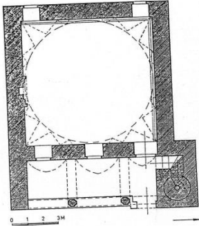
شكل رقم (٤): مسقط أفقي لجامع صرجالي بقونية يمثل طراز الجامع القبة في العمارة السلجوقية (عن: أصلان آبا)
