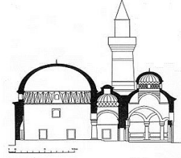
شكل رقم (٧): قطاع رأسي ليشيل جامع في ازنيك يوضح السقيفة المزدوجة الداخلية والأخرى الخارجية به (عن: Goodwin)
