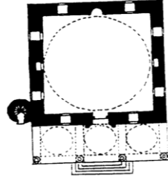
شكل رقم (١٠): مسقط أفقي لجامع فيروز أغا في إستانبول يوضح استمرار طراز بورصة (عن: Archnet)
