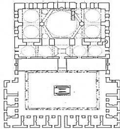
شكل رقم (١٢): مسقط لجامع الأدميرال سنان في بشكطاش في إستانبول يوضح قطاع قبه السداسية (عن: Kuran)
