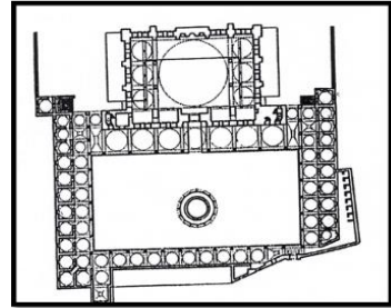
شكل رقم (١١): مسقط أفقي لجامع مهرماه عند أدرنة قابي بإستانبول يوضح قطاع قبته المربع (عن: أصلان آبا)
