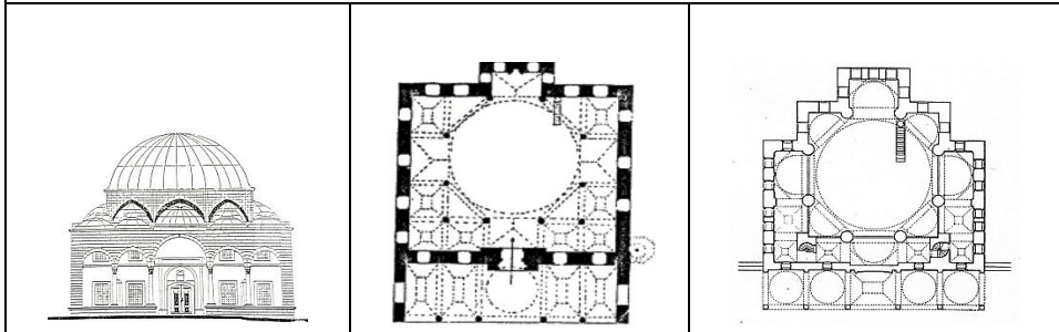
شكل رقم (٣٠): مسقط أفقي وواجهة مسجد ذنجري باليونان يوضح زيادة مساحة مخطظه من خلال محور صليبي وسقيفته الأمامية (عن: أحمد أمين)
