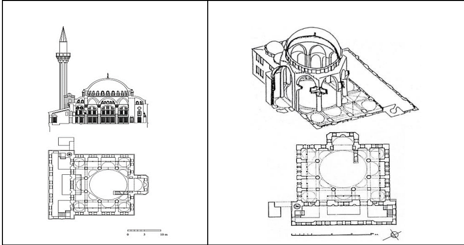
شكل رقم (٢٨): مسقط أفقي ومنظور وقطاع لجامع صوققلو محمد باشا بعزب قابي في إستانبول يوضح زيادة مساحة مخطظه من خلال ثمانية أنصاف قباب بجوانب قبة المئمنة (عن: Kuran)
