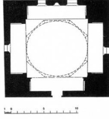
شكل رقم (٨): مسقط أفقي لجامع أورخان في بيلاجيك يوضح زيادة مساحته من خلال ما يشبه أربع دخلات (عن: Goodwin)
