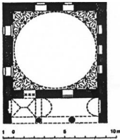
شكل رقم (٦): مسقط لجامع حاجي أوزبك في ازنيك وفق طراز بورصة الأول (عن: Goodwin)
